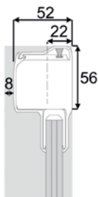
Boîtier 46
