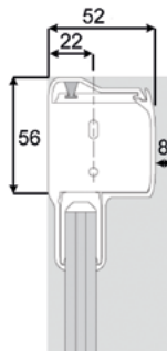
Boîtier 46
