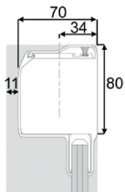
Boîtier 65
