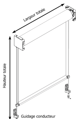
Prise de côtes store toile vertical
