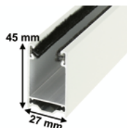
Coulisse pour lame de 13 mm
