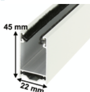
Coulisse pour lame de 8 mm
